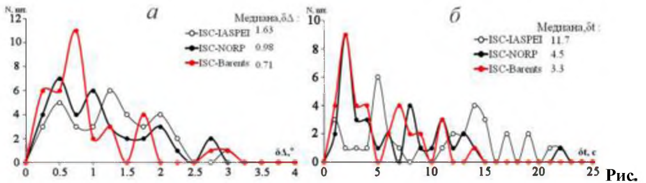
6. Распределение отклонений при определении параметров эпицентров:
