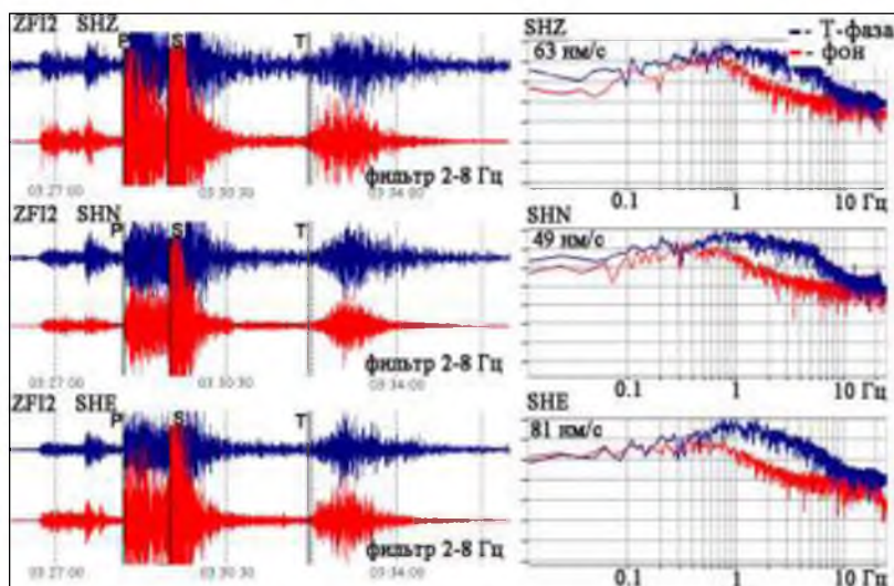
Рис. 8. Пример записи регионального землетрясения на с/с ZFI (26.05.2012 г., район арх. Шпицберген, \varphi=86.04^\circ с.ш., \lambda=30.80^\circ в.д., m_b=5.2 ) и амплитудный спектр Т-фазы в сравнении с микросейсмическим фоном ZFI2 – с/с “Земля Франца-Иосифа-2” SHZ, SHN, SHE – короткопериодные каналы с/с “Земля Франца-Иосифа-2”
